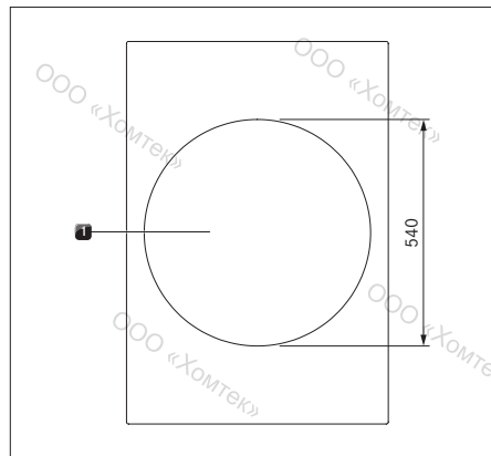
рис. 4.10 Конструкция варочной панели PKIW3 и размер конфорок
