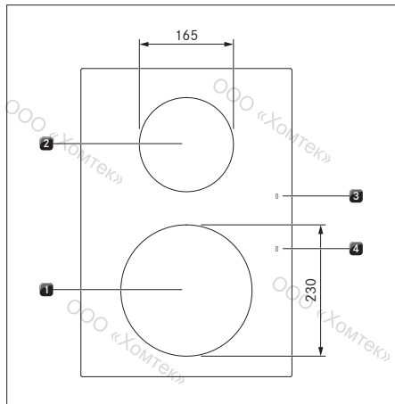
рис. 4.9 Конструкция варочной панели PKI3 и размер конфорок
