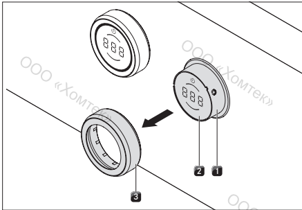
рис. 8.6 Снятие кольца поворотной ручки управления
