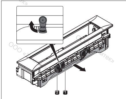
рис. 8.4 Демонтаж поддона для обслуживания
