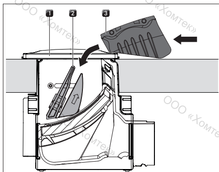
рис. 8.3 Вставка запорного клапана
