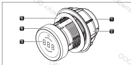
рис. 4.1 Конструкция поворотной ручки управления
