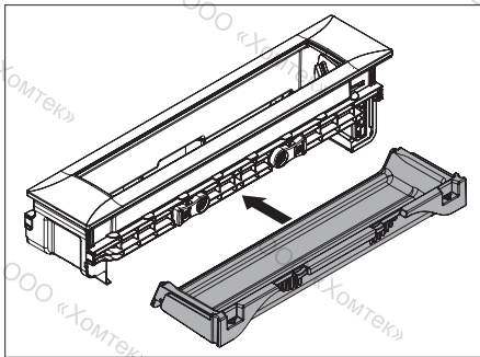
рис. 8.5 Монтаж поддона для обслуживания
