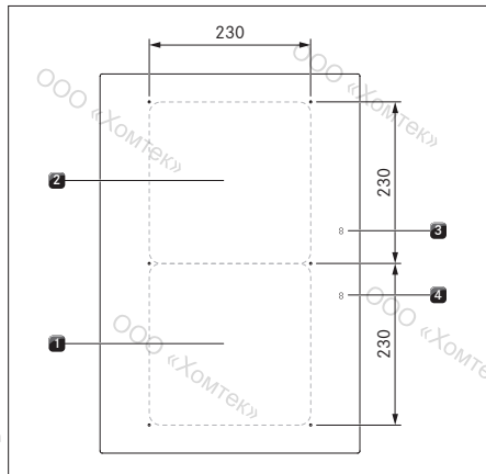
рис. 4.8 Конструкция варочной панели PKF13 и размер конфорок
