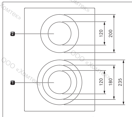
рис. 4.11 Конструкция варочной панели PKC3 и размер конфорок
