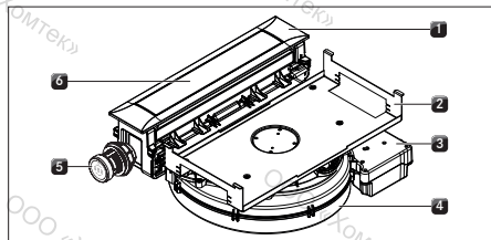
рис. 4.6 Система вытяжки РКАС3/РКАС3AB
