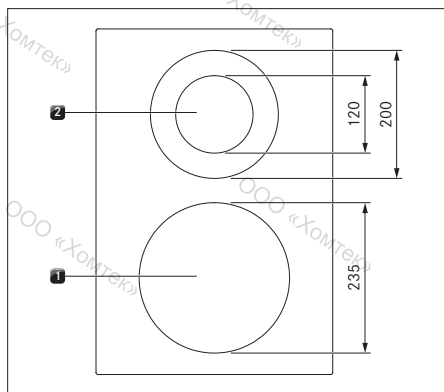
рис. 4.13 Конструкция варочной панели РКНЗ и размер конфорок
