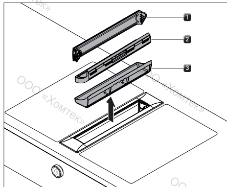
рис. 8.1 Демонтаж компонентов жирового фильтра
