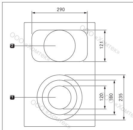
рис. 4.12 Конструкция варочной панели РКВЗ и размер конфорок
