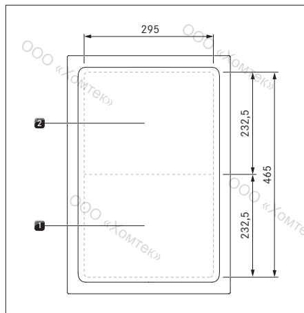
рис. 4.14 Конструкция тэппан-гриля из нержавеющей стали РКТЗ и размер конфорок
