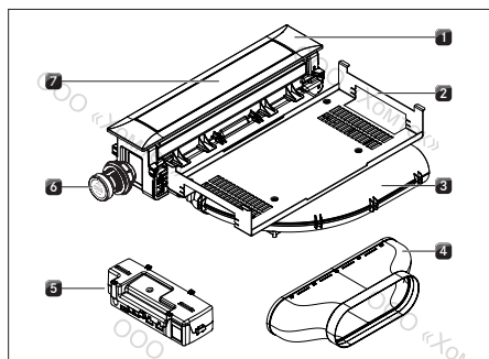
рис. 4.5 Вытяжка РКАЗ/РКАЗAB
